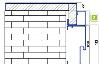
Rysunek techniczny
