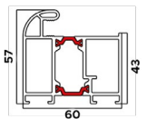
Rysunek techniczny
