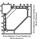
Rysunek techniczny
