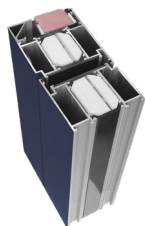
Przekrój drzwi ALU Fireline
